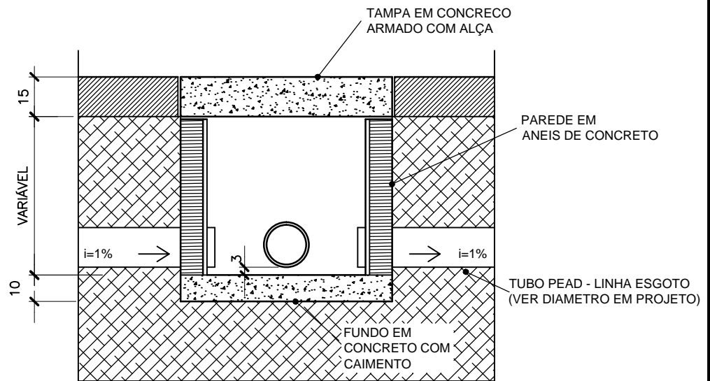
CAIXA DE INSPEÇÃO D60cm CORTE - ESCALA 1/20
