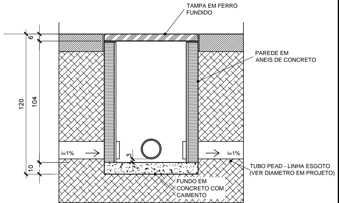
POÇO DE VISITA D60cm PLANTA BAIXA - ESCALA 1/20
