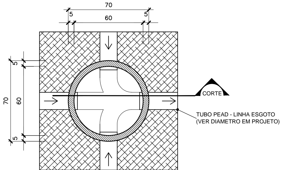
POÇO DE VISITA D60cm PLANTA BAIXA - ESCALA 1/20
