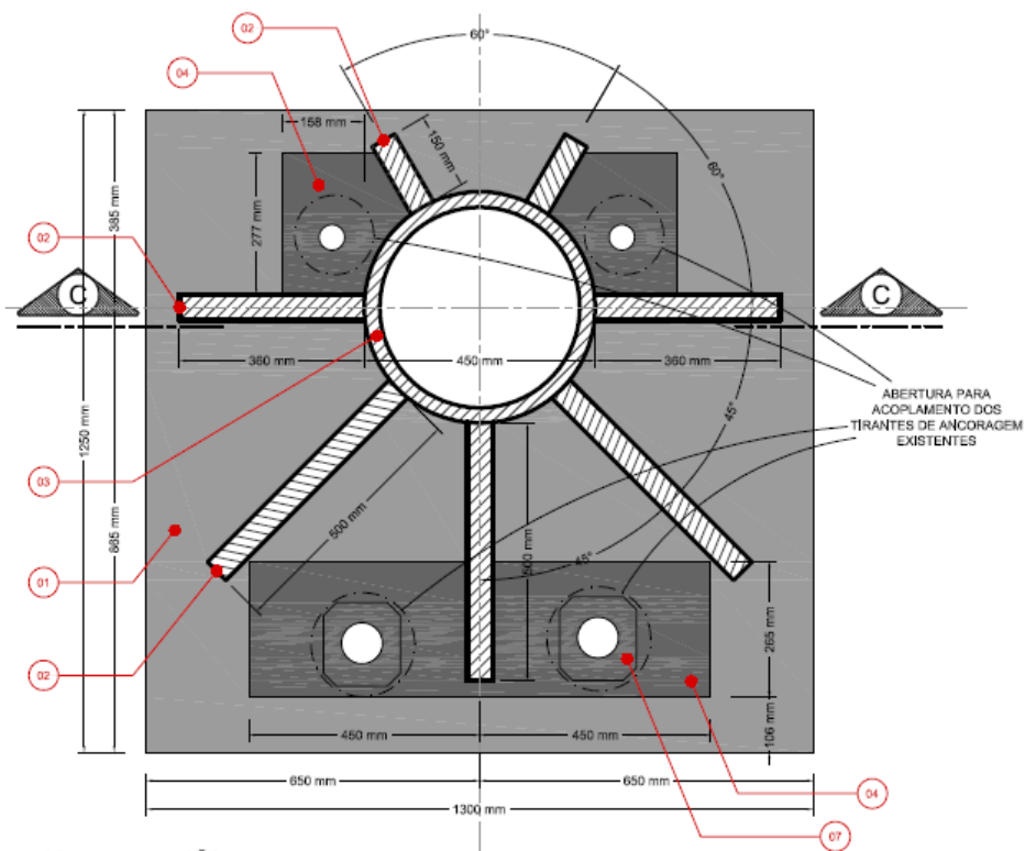
CABEÇO DE AMARRAÇÃO DETALHES CONSTRUTIVOS Seção Horizontal ESCALA: 1:10
