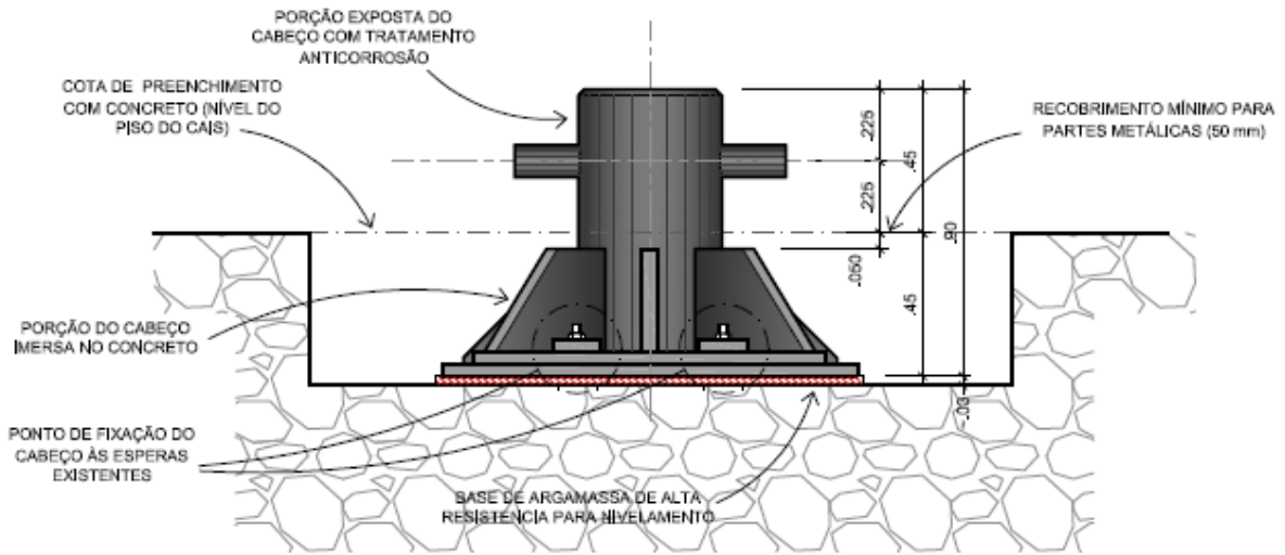
CABEÇO DE AMARRAÇÃO DETALHES EXECUTIVOS SEÇÃO LONGITUDINAL "A-A"
