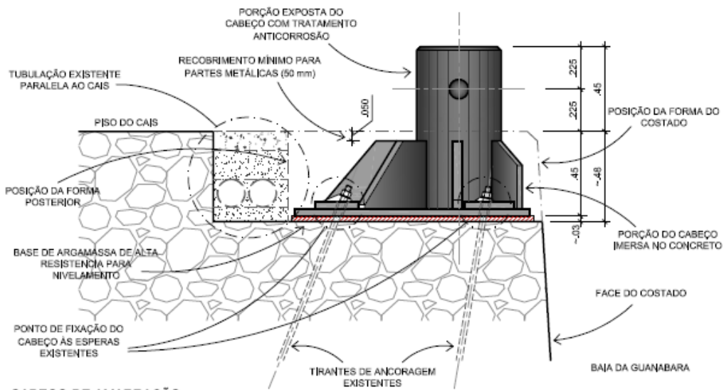
CABEÇO DE AMARRAÇÃO DETALHES EXECUTIVOS SEÇÃO TRANSVERSAL "B-B"
